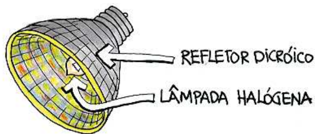
Figura 8-4: Lâmpada halógena e refletor dicróico
