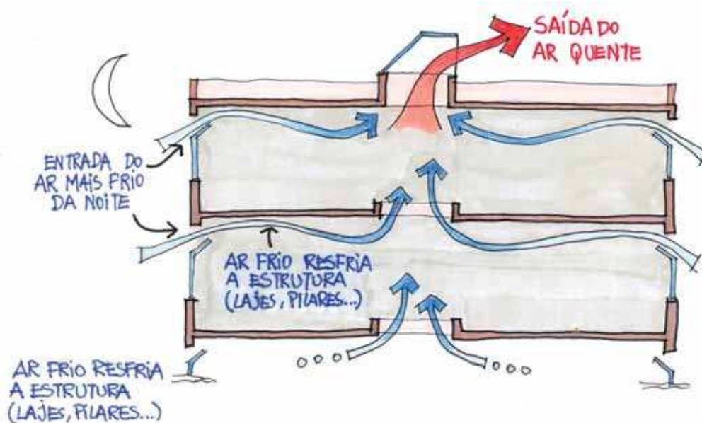
Figura 6-20: Ventilação noturna
