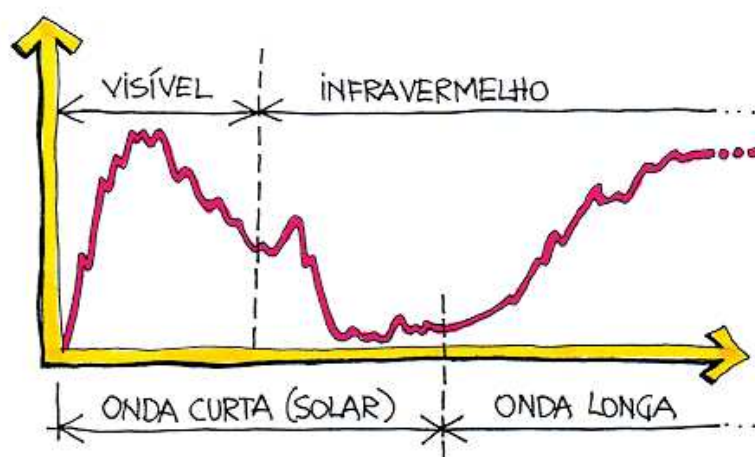
Figura 7-8: Espectro solar
